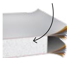
Izolowana ściana boczna / panel drzwiowy Element warstwowy z rdzeniem polistyrenowym 40 mm (EPS W20)
