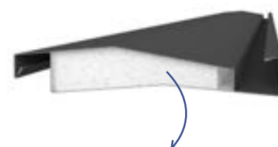
Lamellenstructuur Sandwichconstructie met Peripor-kern
