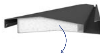
Struttura a lamelle Costruzione a sandwich con anima in Peripor
